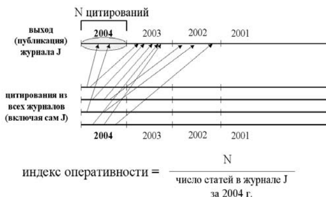
Рис. 4. Вычисление индекса оперативности за 2004 г.
