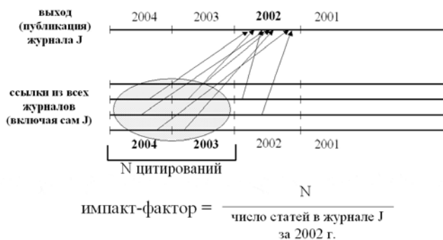
Рис. 3. Вычисление диахронного импакт-фактора за 2002 г.
